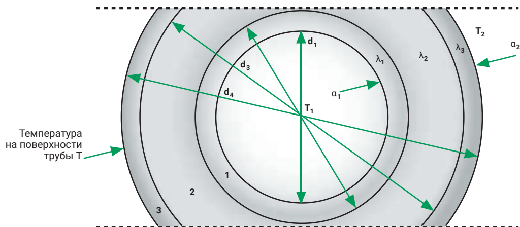
Рис. 5: Потери тепла через трубу при длине трубы 1 метр
