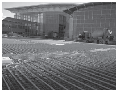
Системы снеготаяния USYSTEMS
