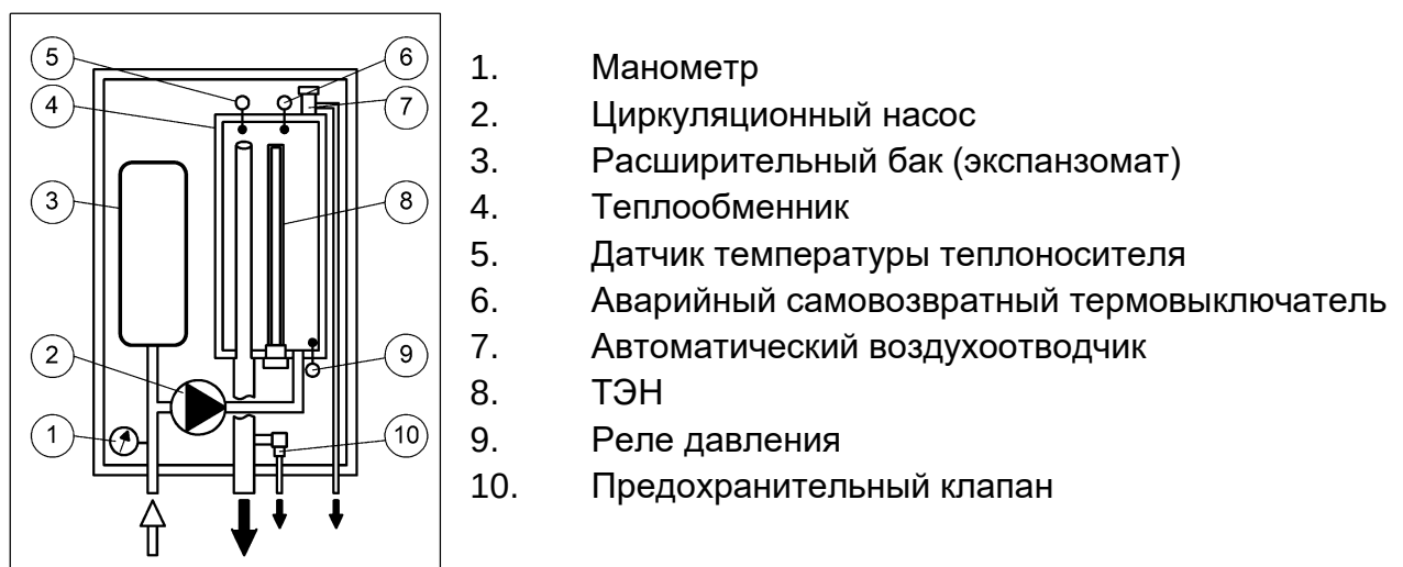
Рисунок 1. Принципиальная схема котла
