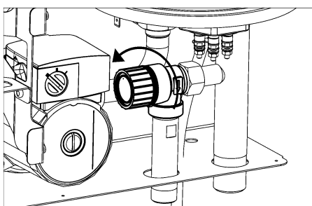
Рисунок 16. Поворот крышки клапана
