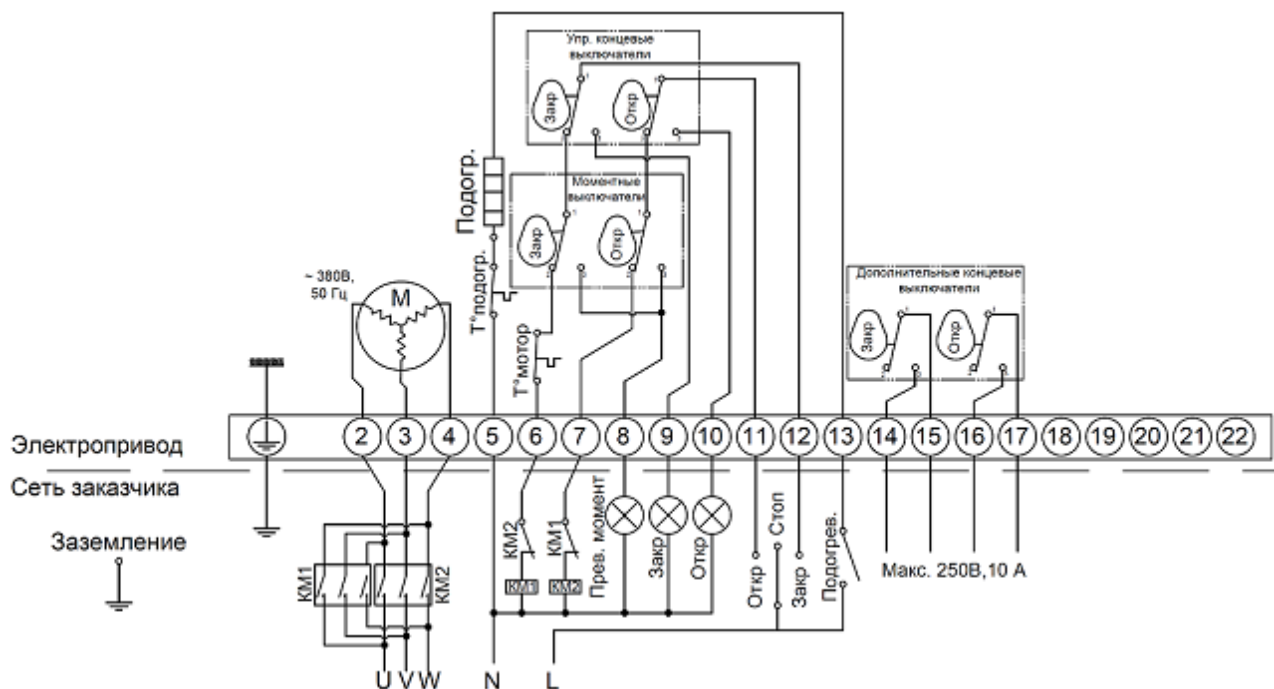
Рис. 3 - Электрические присоединения
