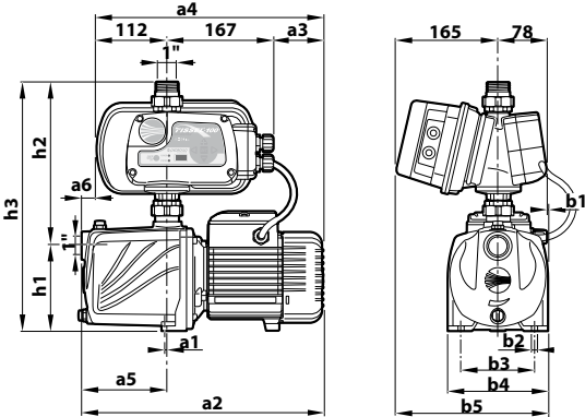
TS1-4CP 100
