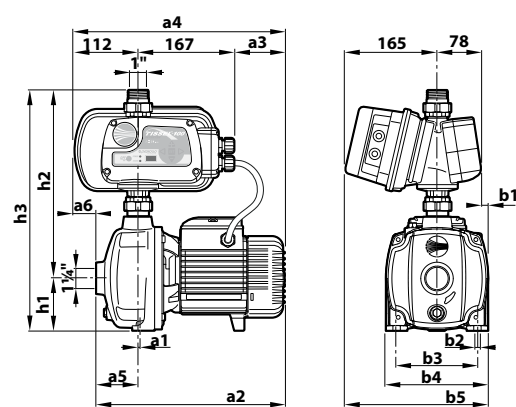
TS1-2CP 25/130
