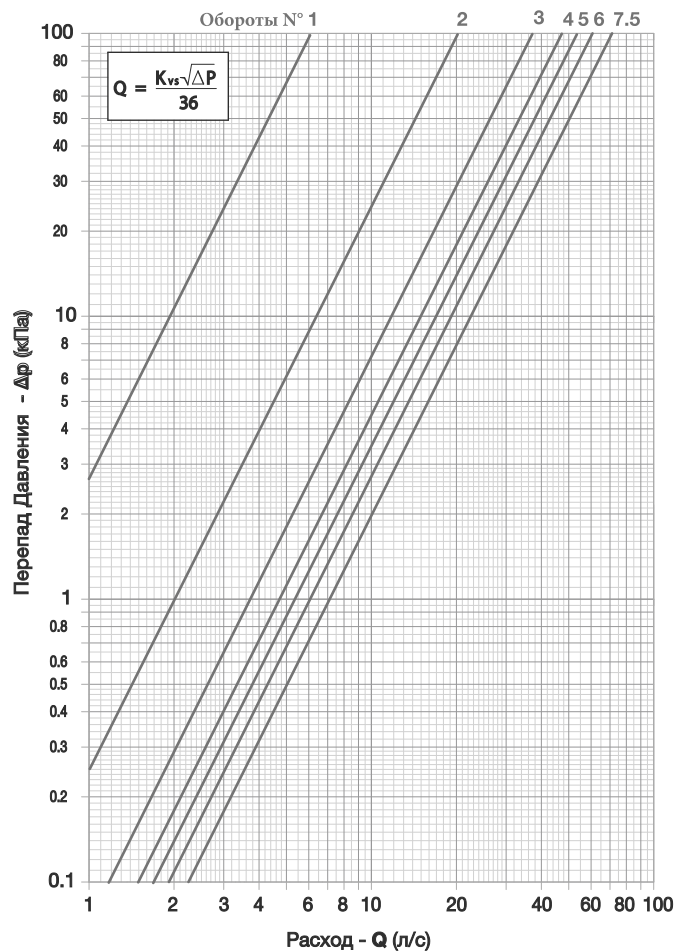
Kv-Kvs (расход в м³/ч при перепаде давления 1 бар)
