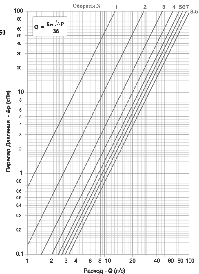
Kv-Kvs (расход в м³/ч при перепаде давления 1 бар)
