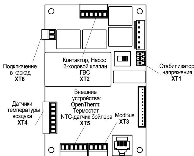
Рисунок 8. Основные разъёмы платы контроллера
