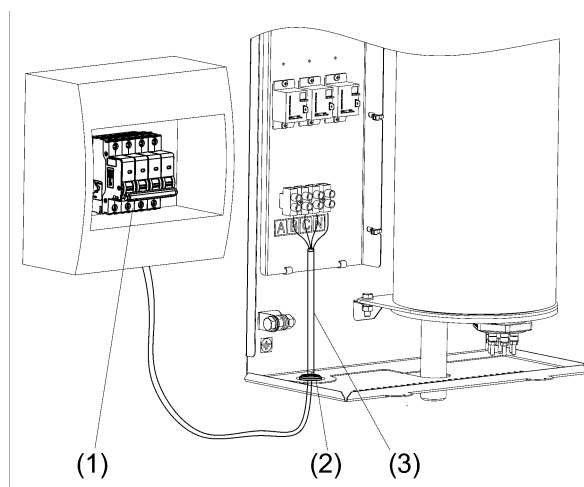
Рисунок 7. Подключение котла к электросети
