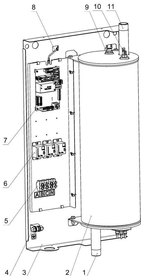
Рисунок 1. Принципиальная схема котла
