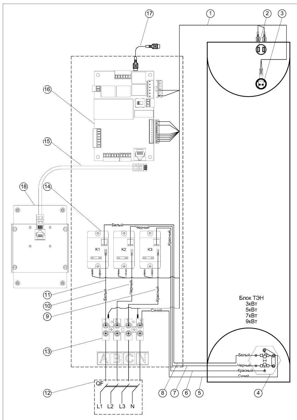
Рисунок 15. Электромонтажная схема подключения EVAN NEXT PLUS-3...9 к сети 380В
