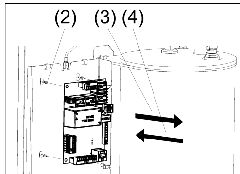
Рисунок 12. Замена платы контроллера
