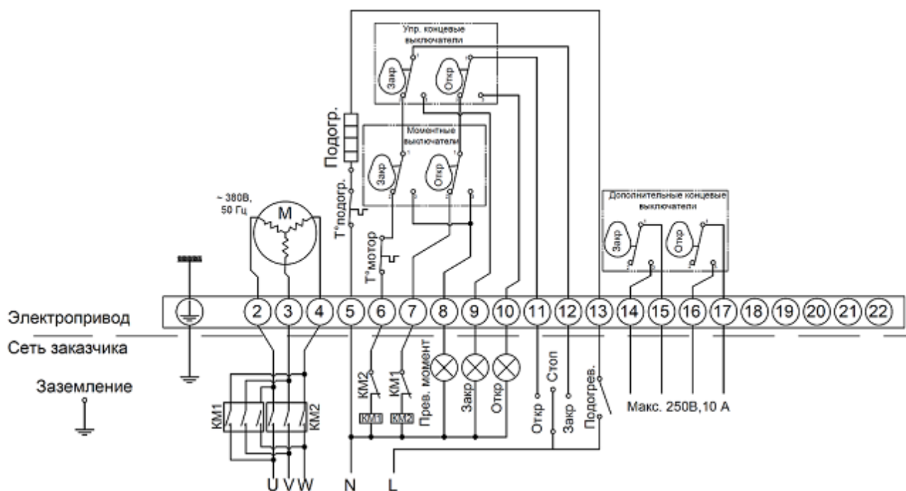
Рис. 3 - Электрические присоединения
